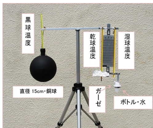
図 1. August 乾湿計と黒球温度計（直径 15cm）による WBGT の測定
